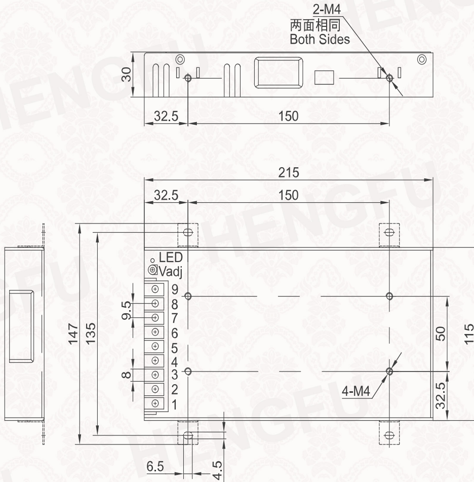
机壳 Frame
